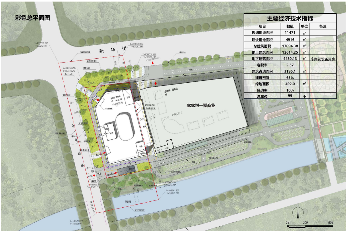
总平面图
