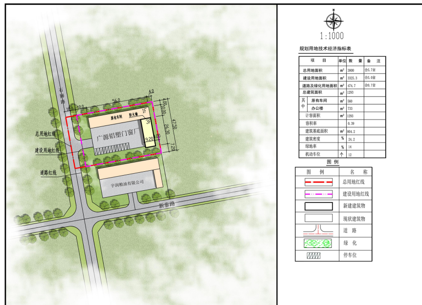
总平面图
